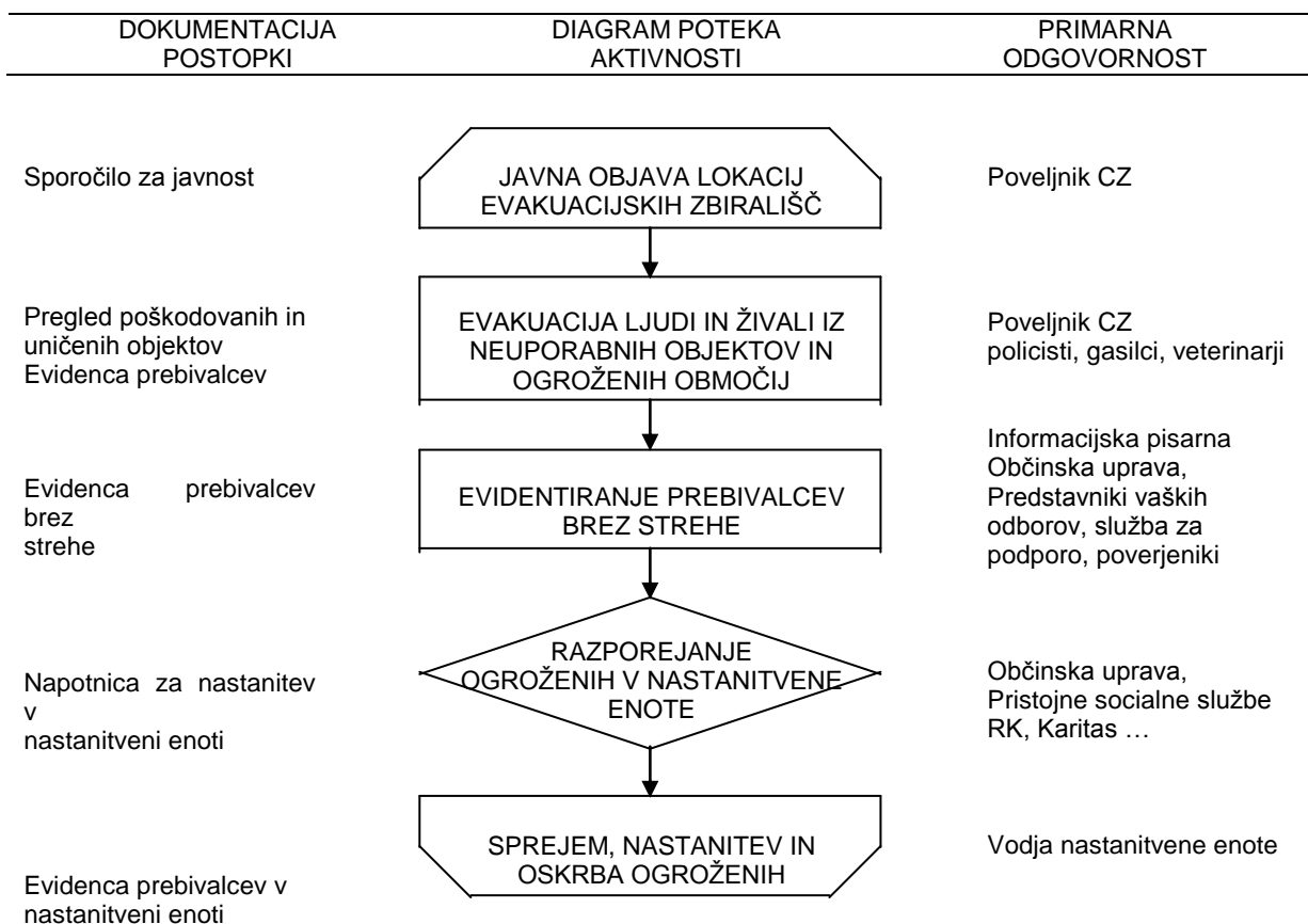
Slika: Shema izvajanja ukrepov evakuacije ob nesreči zrakoplova
