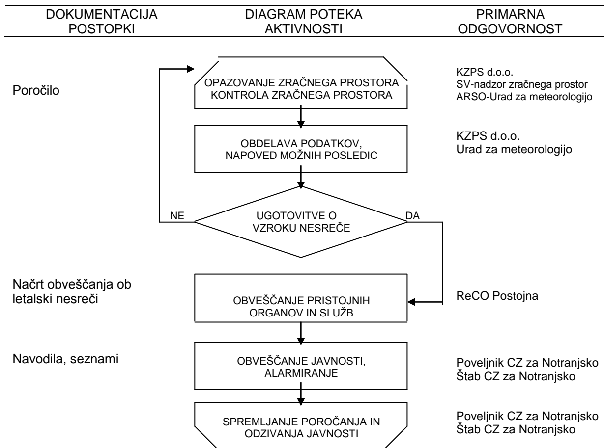
Slika: Shema opazovanja ob nesreči zrakoplova
