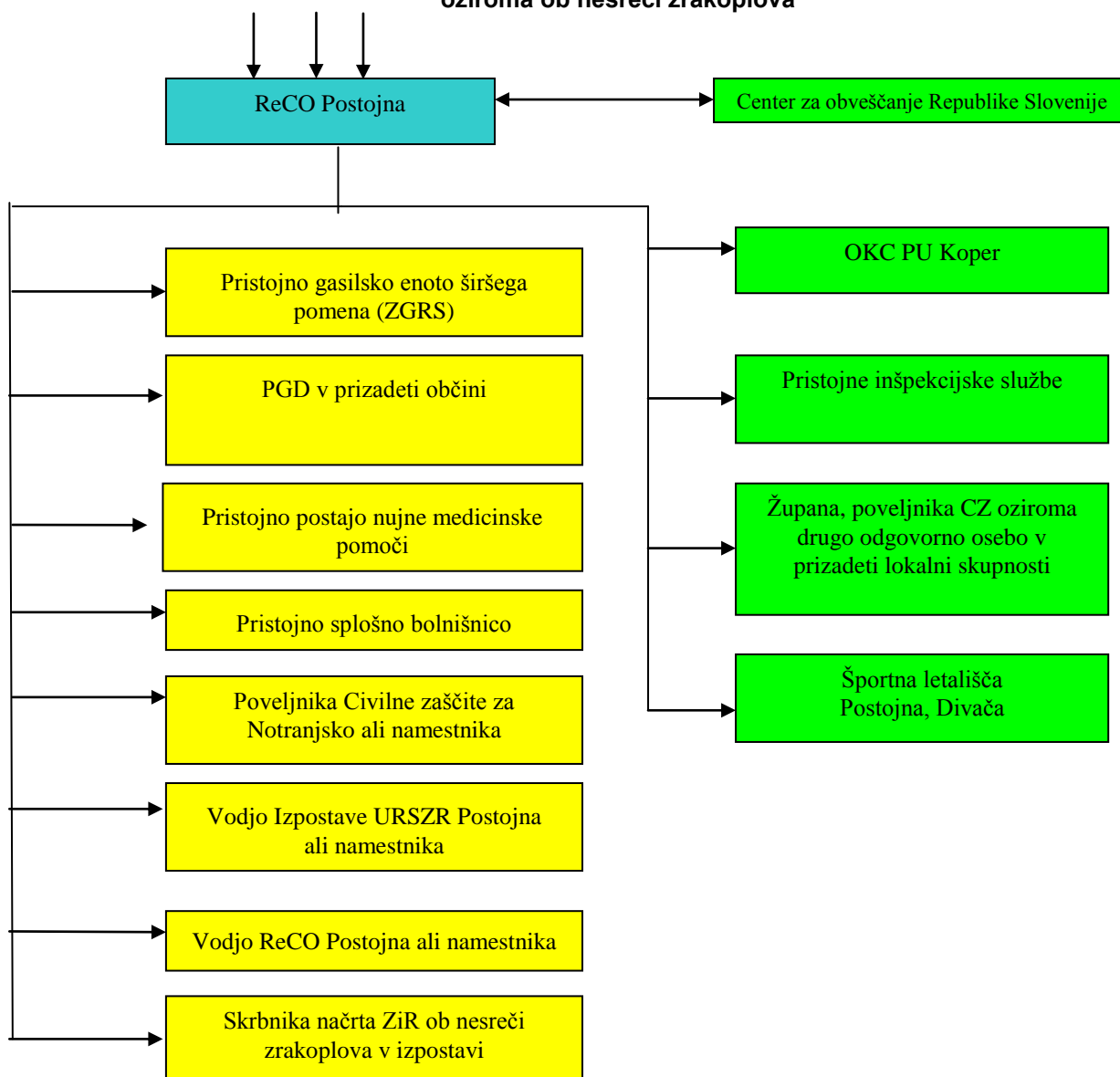
Slika: Shema obveščanja Regijskega centra za obveščanje Postojna v primeru zrakoplova v sili oziroma ob nesreči zrakoplova
